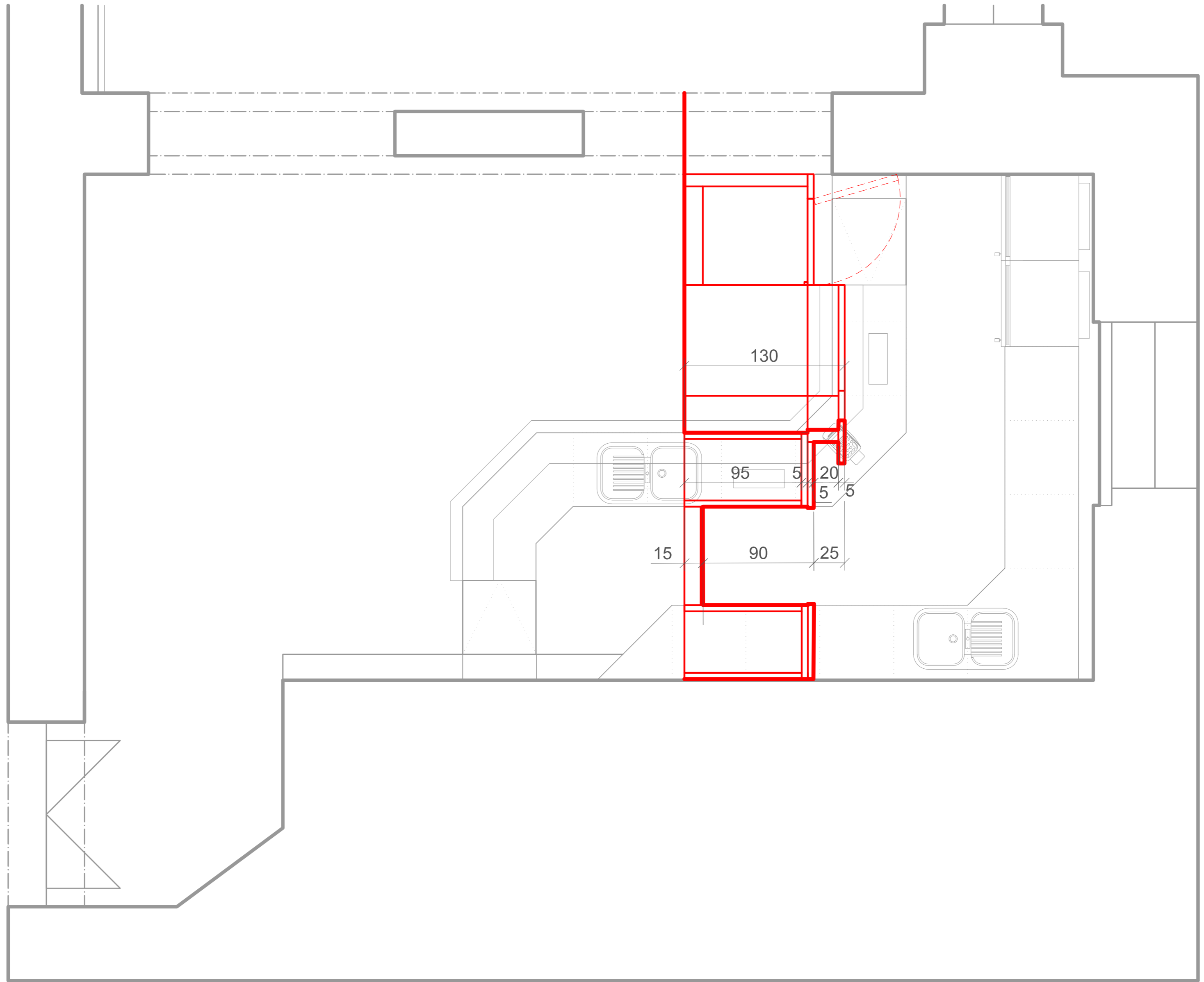
Sklopený rez - Bar
