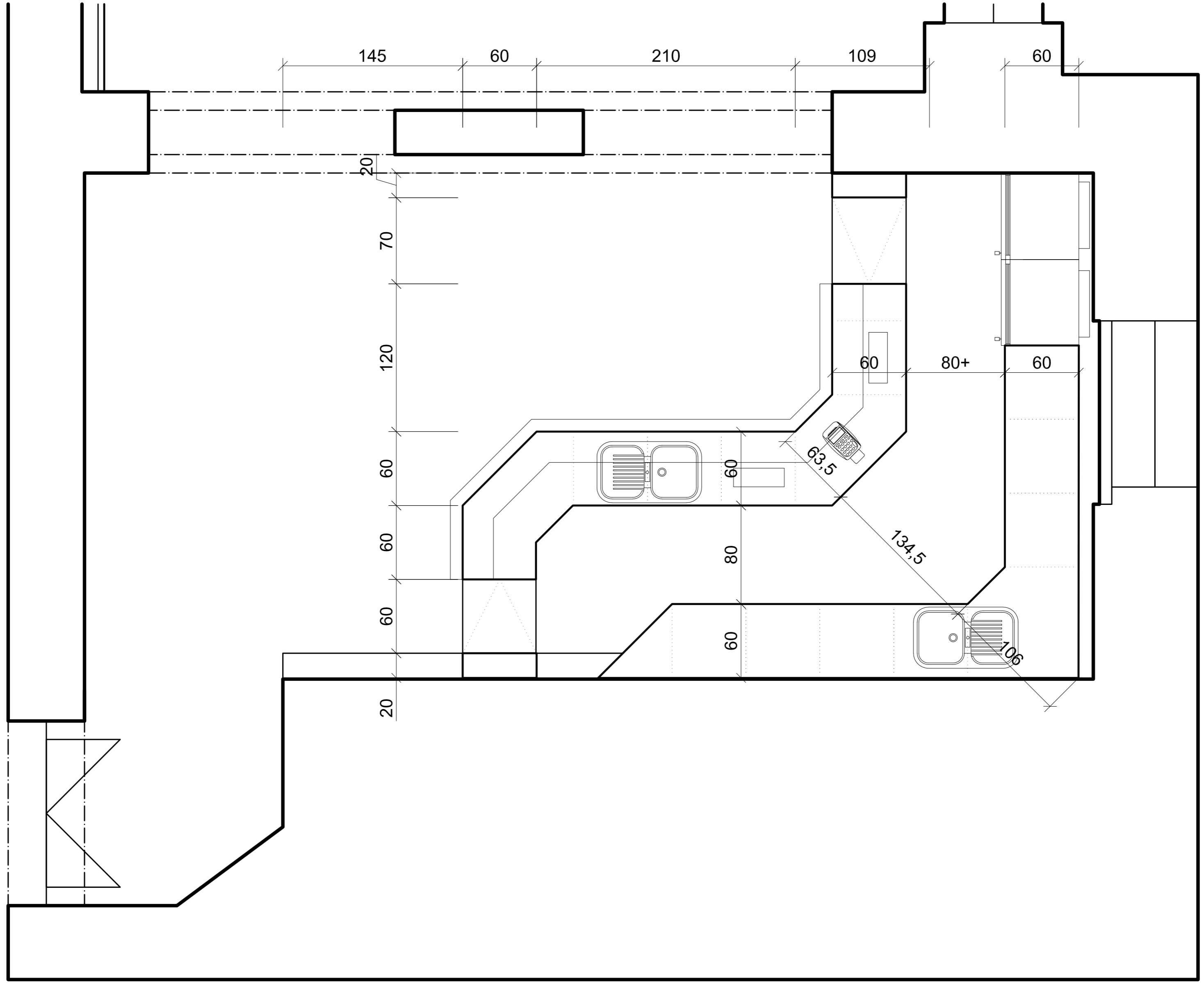
Pôdorys - Bar
